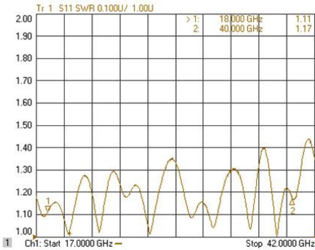
1. 输入驻波比 Input VSWR
