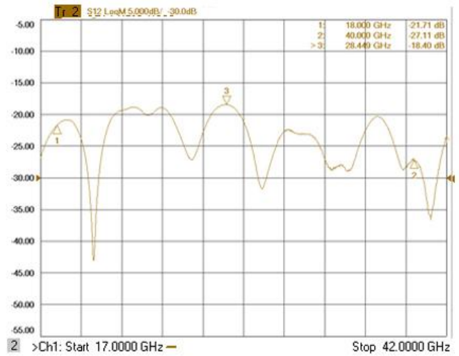
2. 隔离度 Isolation
